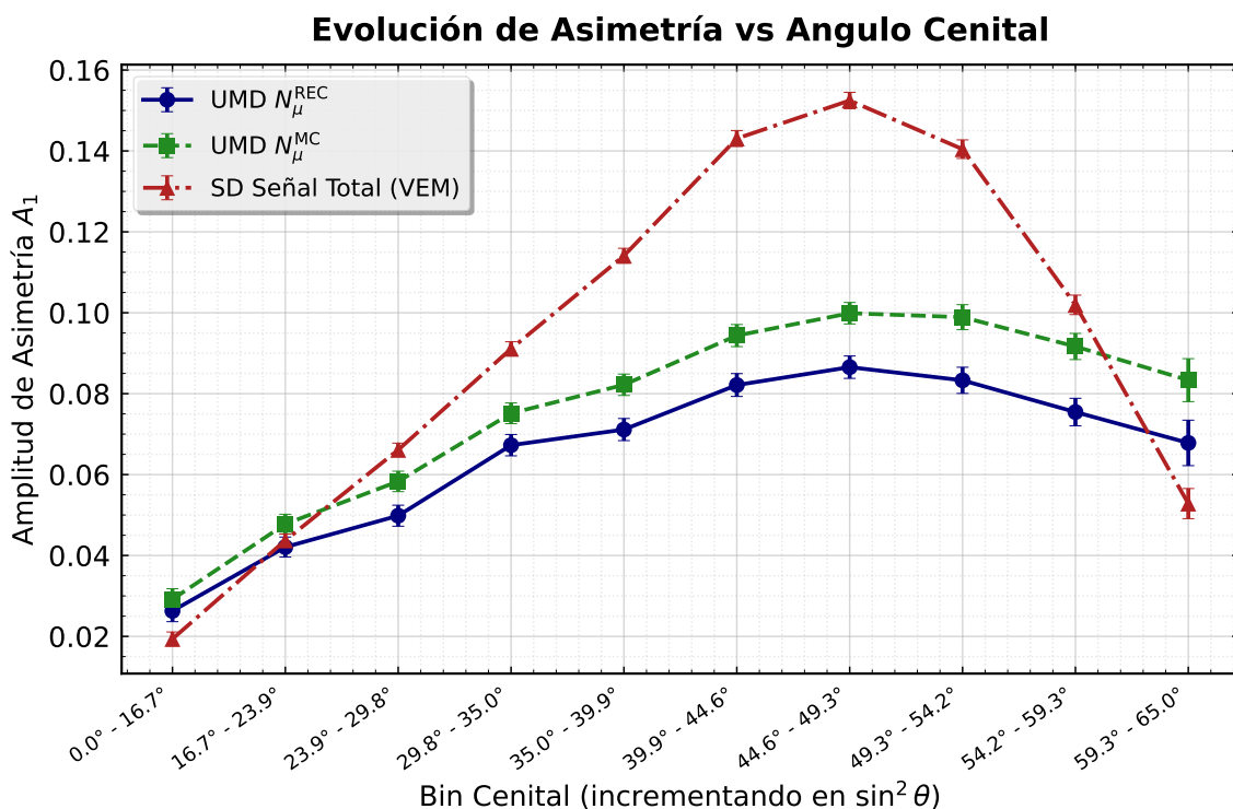
Figura 5.2: Evolución de la amplitud A_1 con su error en función de \theta para el UMD (REC en azul, MC en verde) y el SD (rojo). Se observa la inversión de dominancia entre el SD y el UMD a altas inclinaciones.
