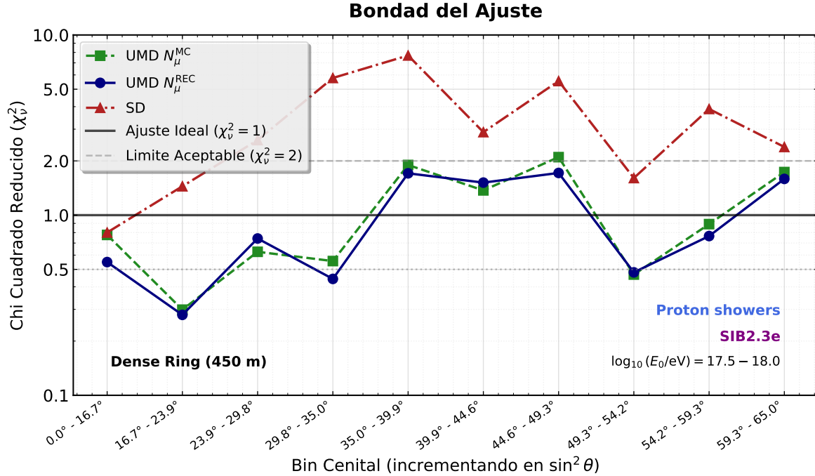
Figura 5.3: Bondad de ajuste \chi^2_v para los bins cenitales. Se observa que los ajustes del UMD (REC y MC) se mantienen cercanos a la unidad, mientras que el SD presenta valores elevados debido a la alta precisión estadística de la muestra.
