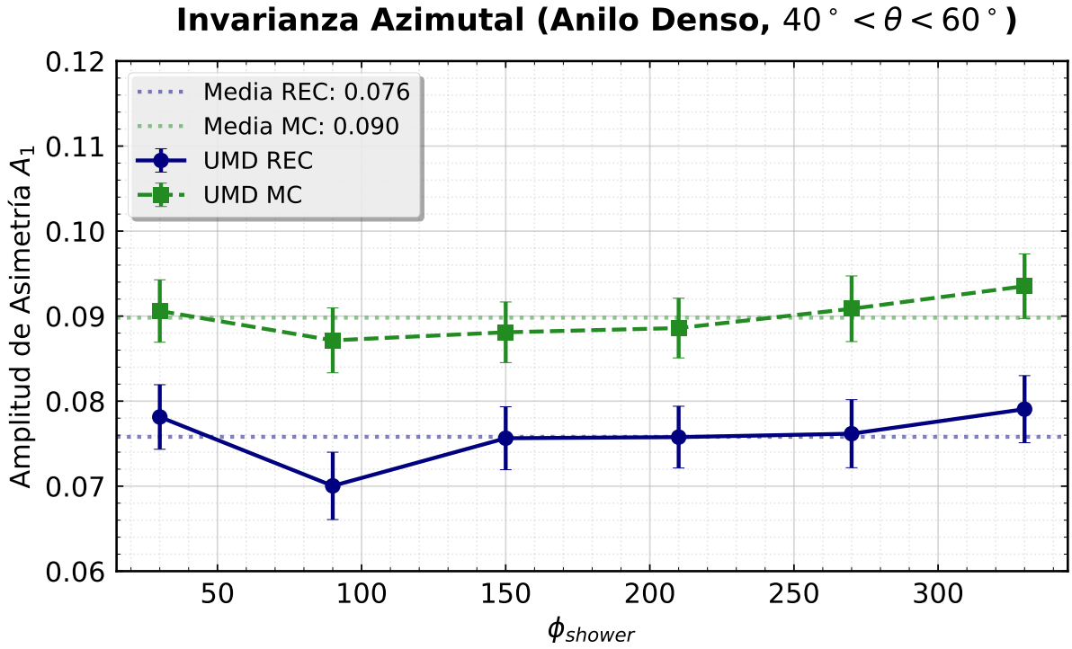
Figura 5.7: Amplitud A_1 en función del ángulo azimutal de la lluvia. Se observa la independencia del observable respecto a la dirección de arribo.
